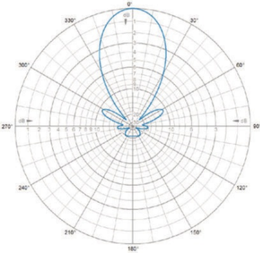
H-Plane | 405 MHz
