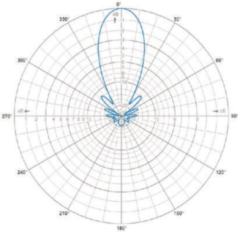
H-Plane | 405 MHz
