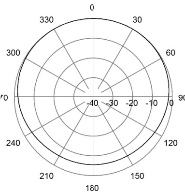
H-Plane | 158 MHz
