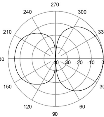
E-Plane | 158 MHz
