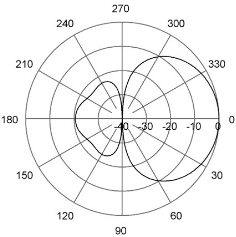
E-Plane | 154 MHz
