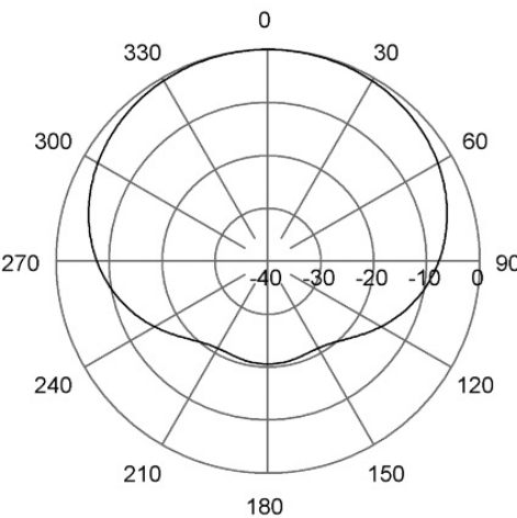
H-Plane | 154 MHz
