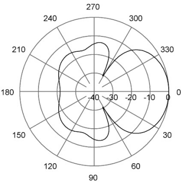
H-Plane | 390 MHz
