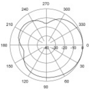
E-Plane | 390 MHz
