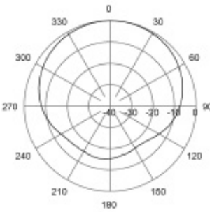
H-Plane | 390 MHz
