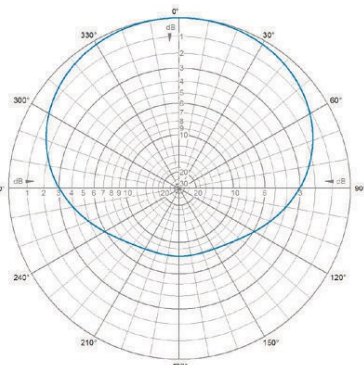
H-Plane | 405 MHz | 0°
