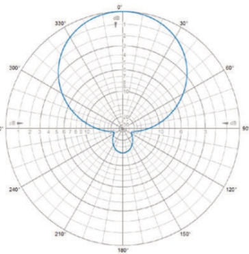
H-Plane | 71 MHz
