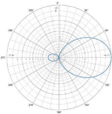
E-Plane | 71 MHz
