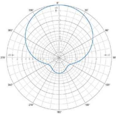
H-Plane | 72 MHz
