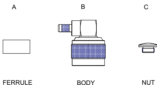
FERRULE
